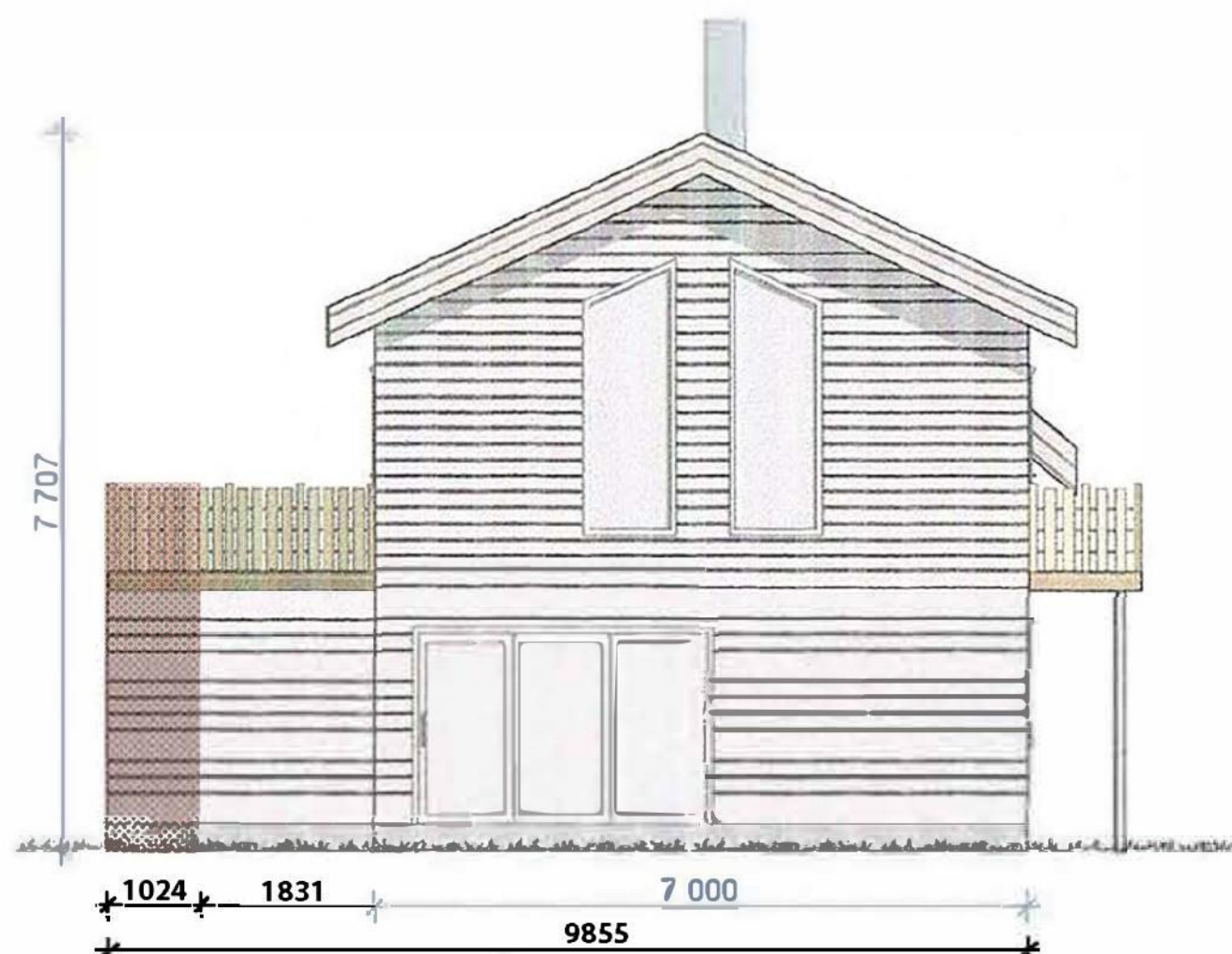
Fasade Øst 1:100
