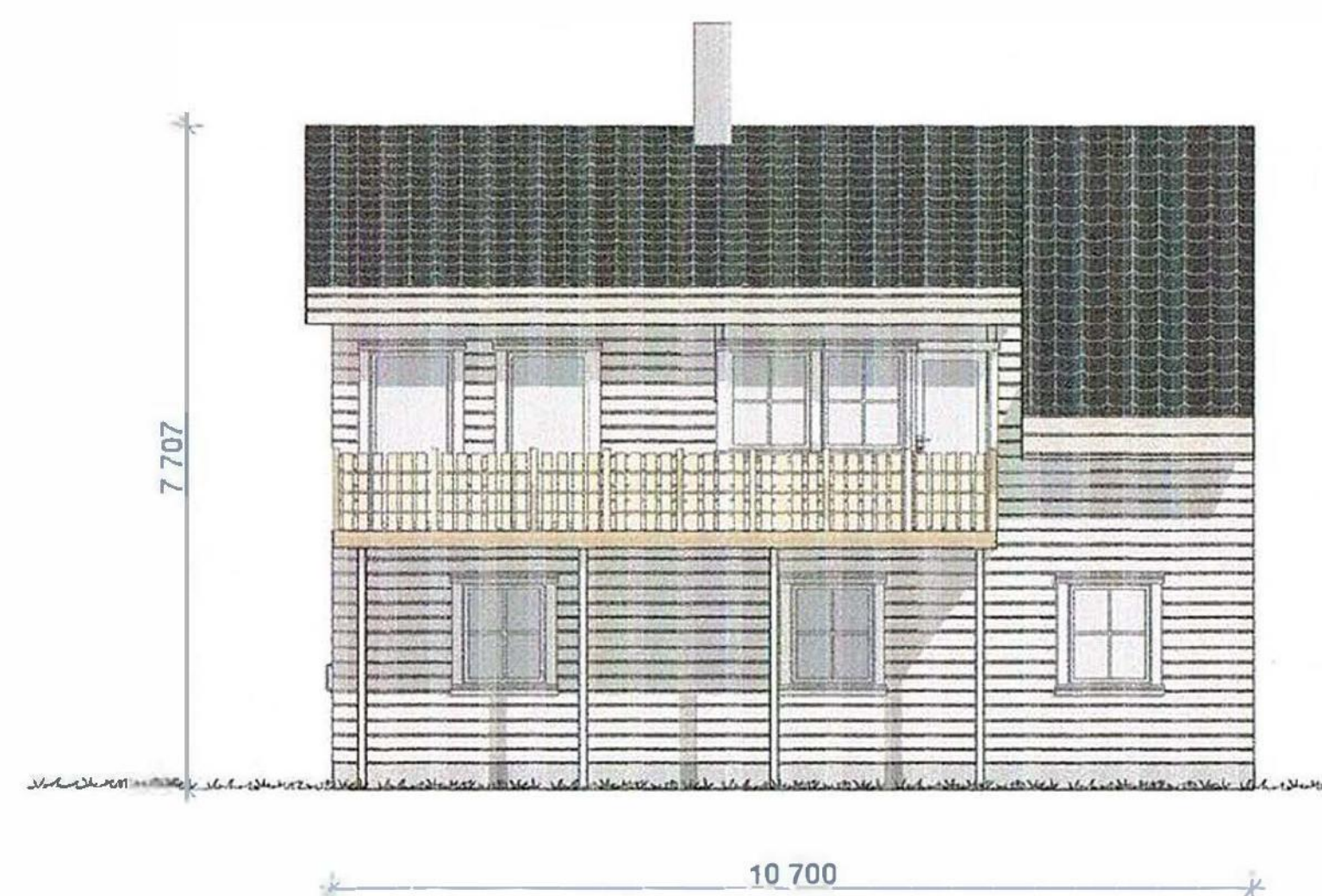
Fasade Nord 1:100
